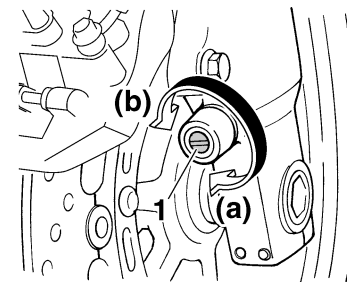
1. Druckstufendämpfungs-Einstellschraube
