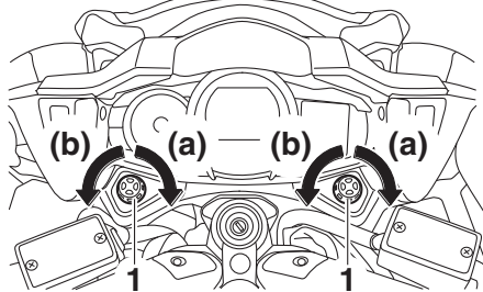
1. Scheinwerferkegel-Einstellknopf
